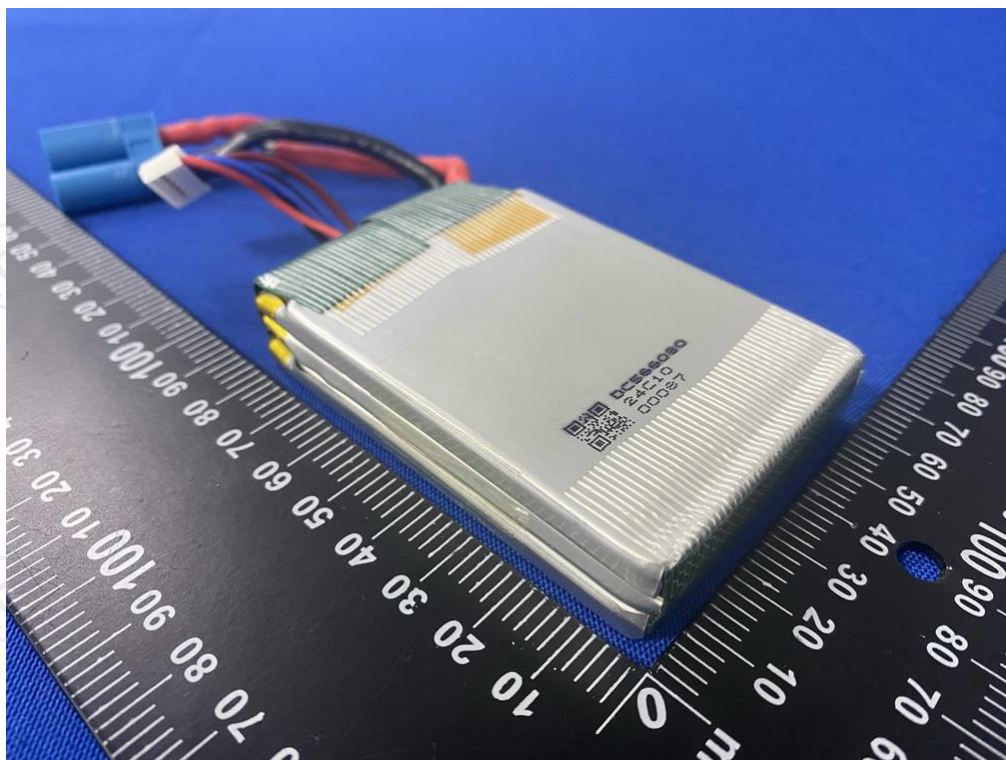
Picture 5. Back view of cell 图片 5. 电芯后视图
