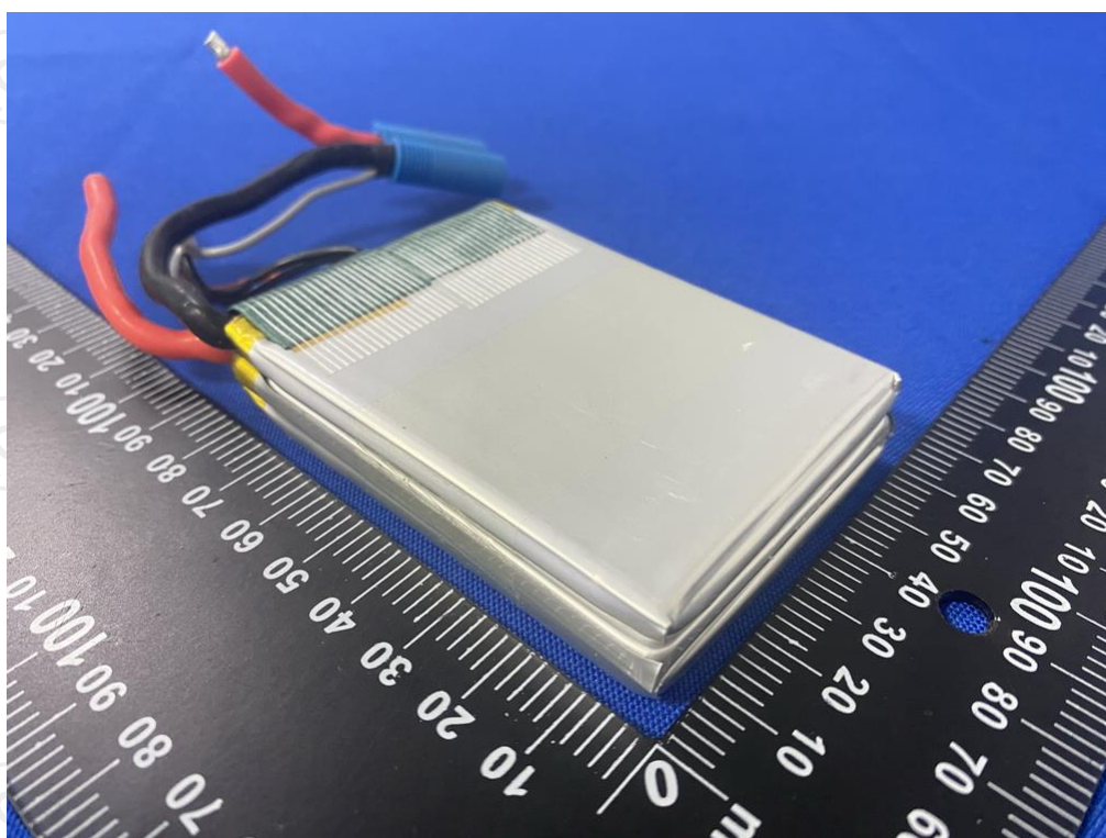
Picture 6. Back view of cell 图片 6. 电芯后视图
